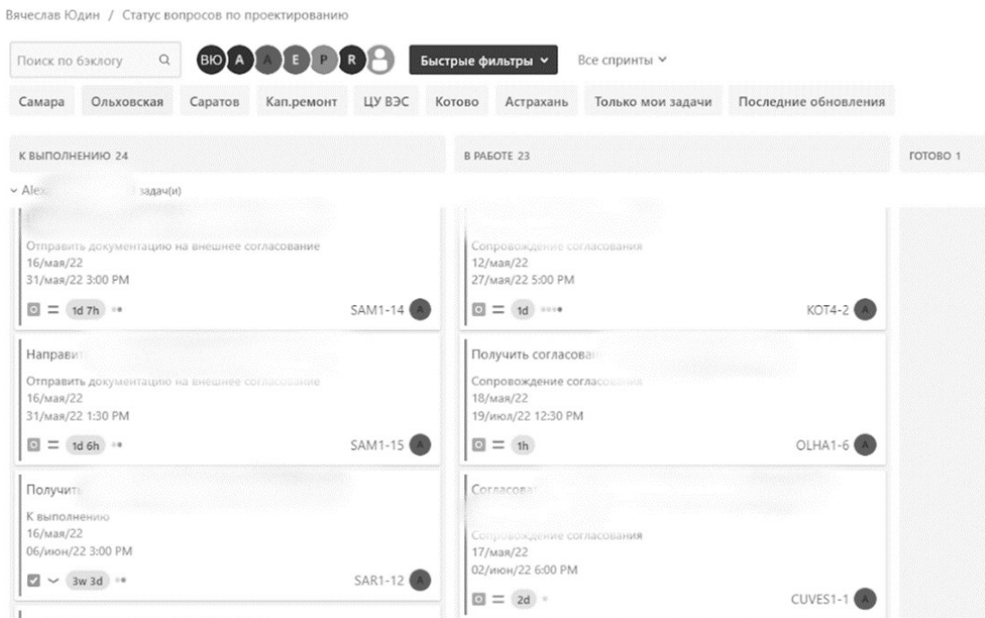
Рисунок 1. Доска Kanban 6
